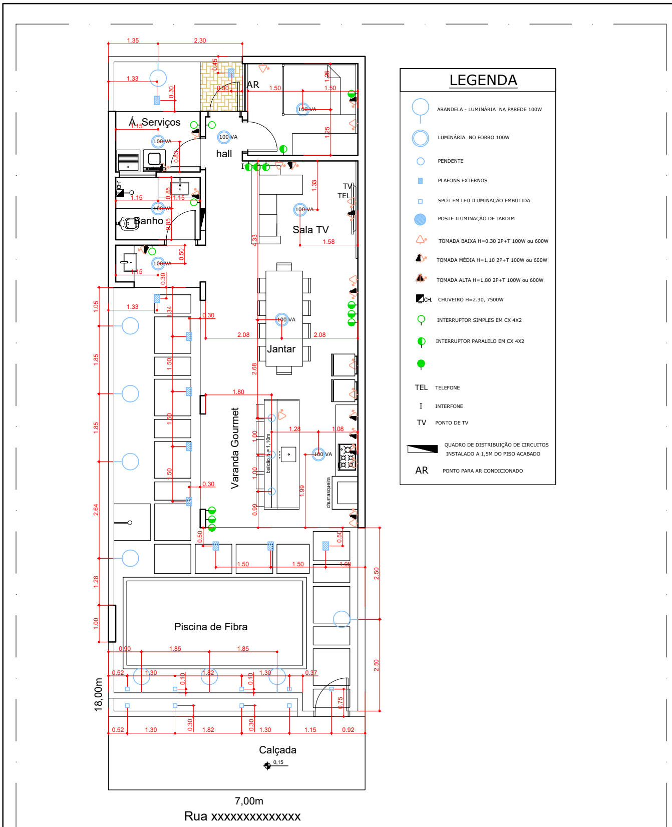
Planta de Pontos Elétricos e Luminárias
